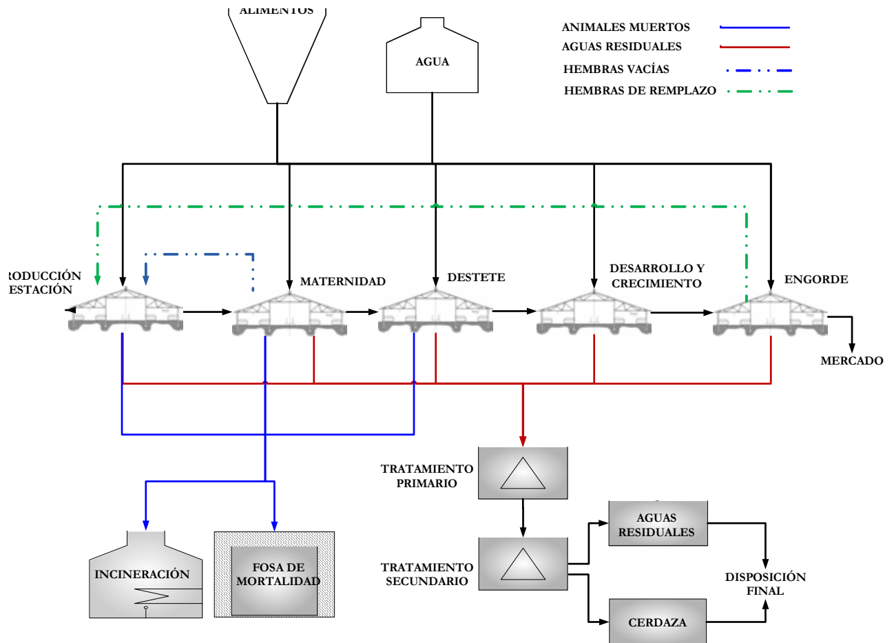
Figura 1. Diagrama de flujo típico de una granja dedicada a la producción de cerdos.
