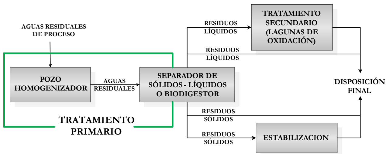
Figura 2. Esquema de un sistema de tratamiento primario y secundario
