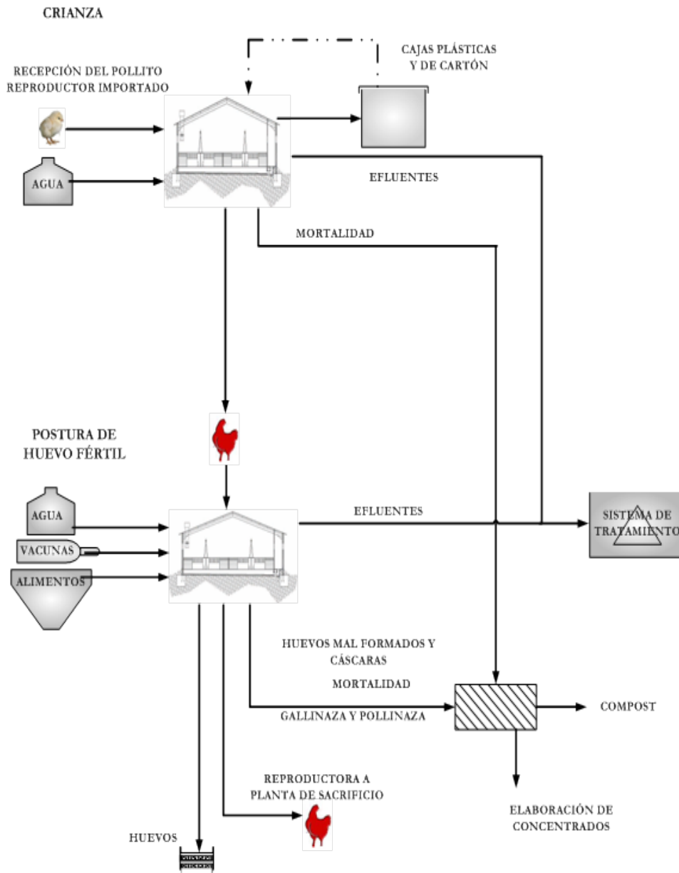
Figura 1. Diagrama de flujo típico de una granja de aves reproductoras.
