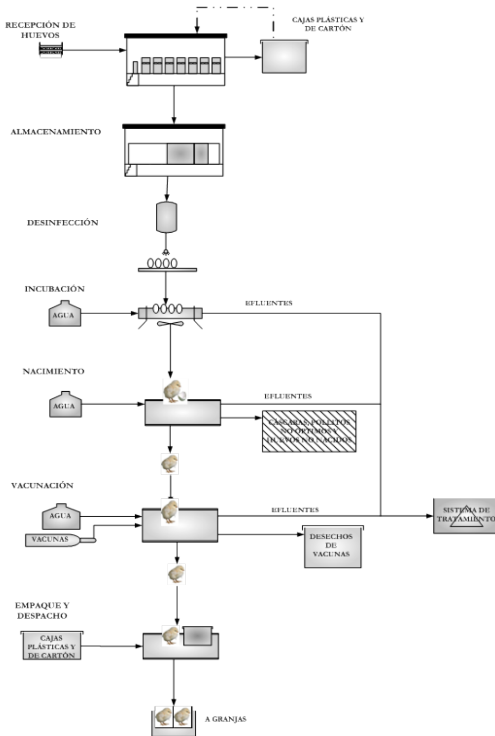
Figura 4 Diagrama de flujo típico de plantas de incubación.
